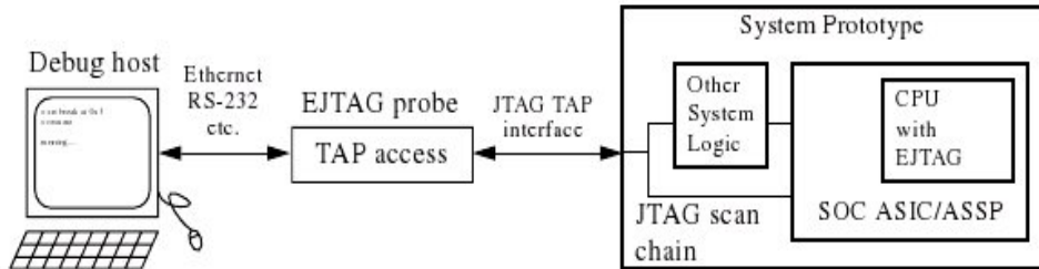
Figure 1: ejtag连接图
